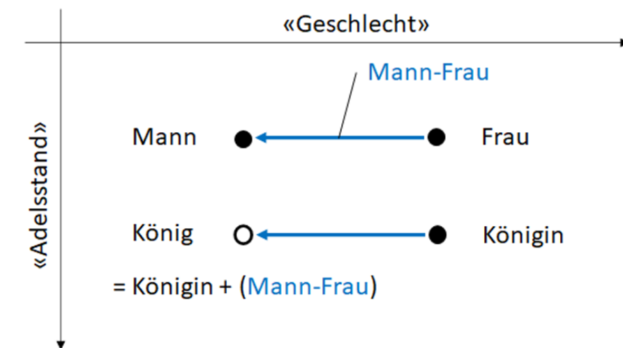
Abbildung 2. Wortraum
